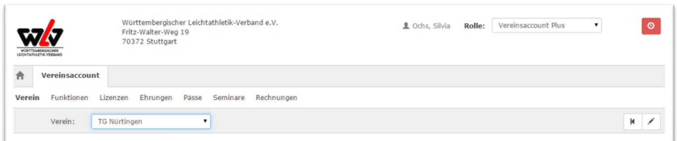
Abbildung 3: Vereinsaccount Module
